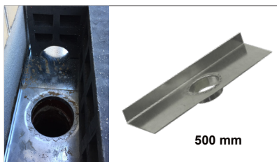
Afløbselement
