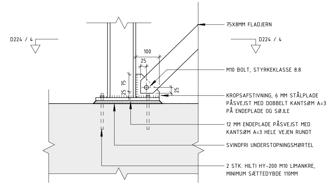
3 SAMLINGSDETALJE I BUND, LODRET SNIT
