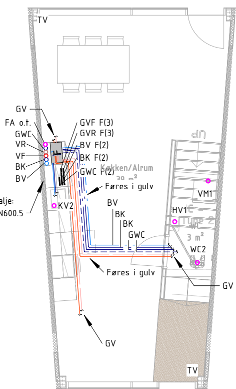
VVS ETAGE 00 Type R-3-A
