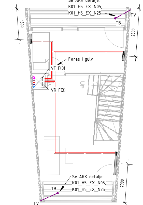
VVS ETAGE 01 Type R-3-E
