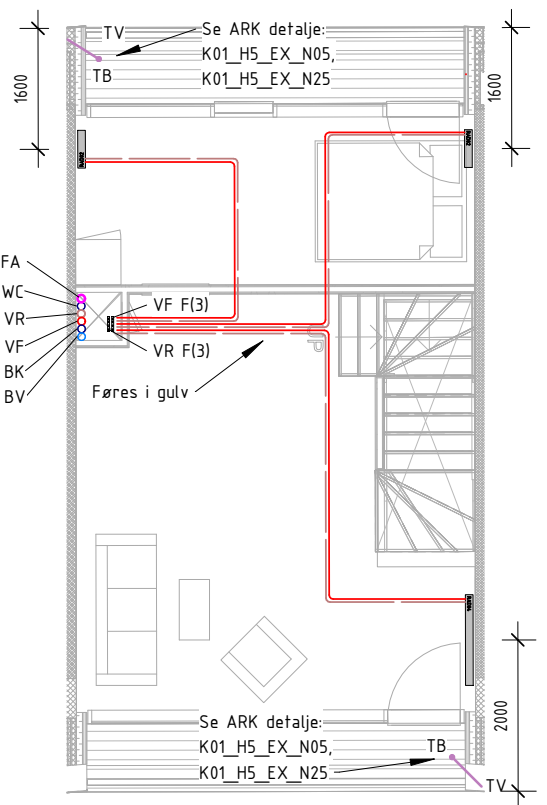
VVS ETAGE 01 Type R-3-C
