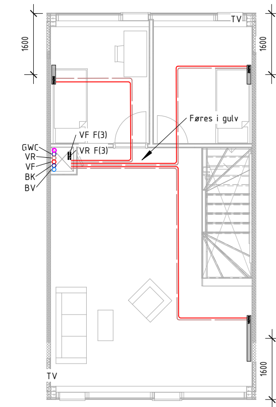
VVS ETAGE 01 Type R-3-D
