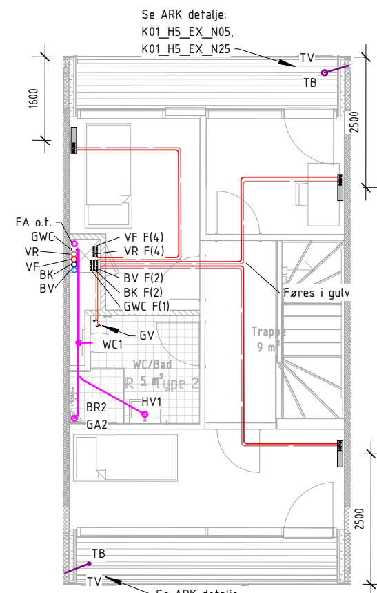
VVS ETAGE 02 Type R-3-D
