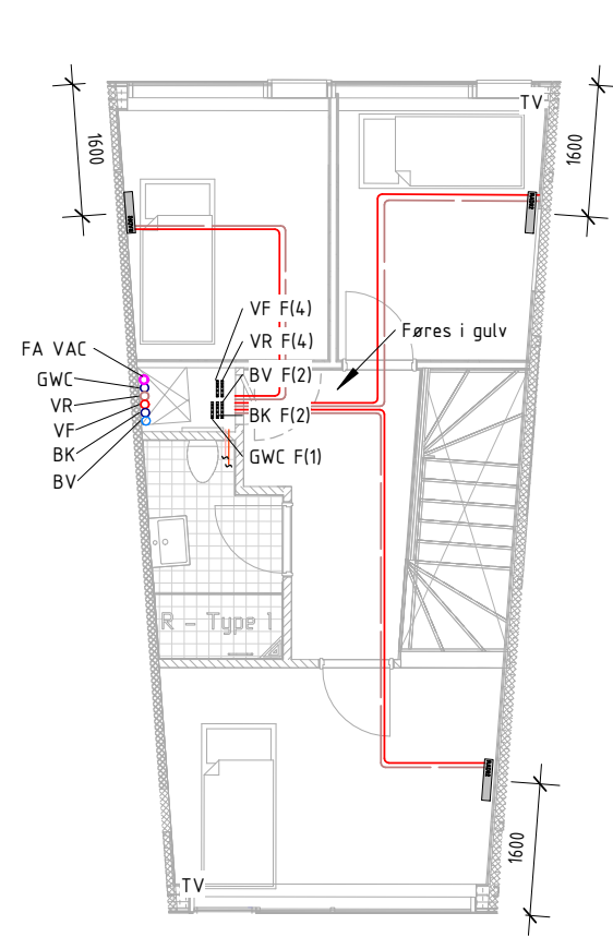
VVS ETAGE 02 Type R-3-E
