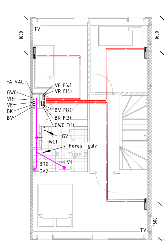
VVS ETAGE 02 - Type R-3-G
