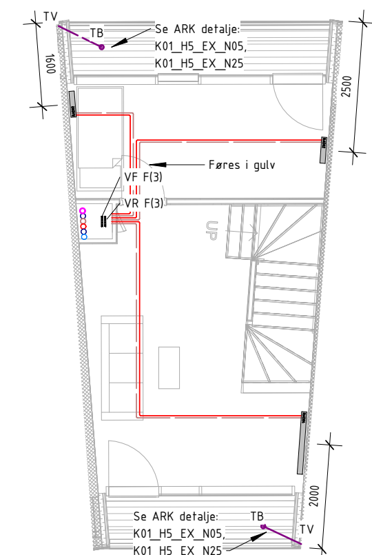
VVS ETAGE 01 Type R-3-F
