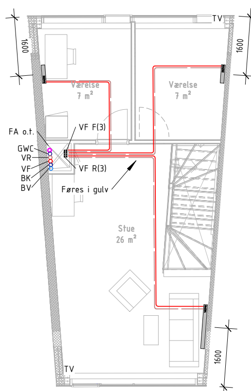
VVS ETAGE 01 Type R-3-B
