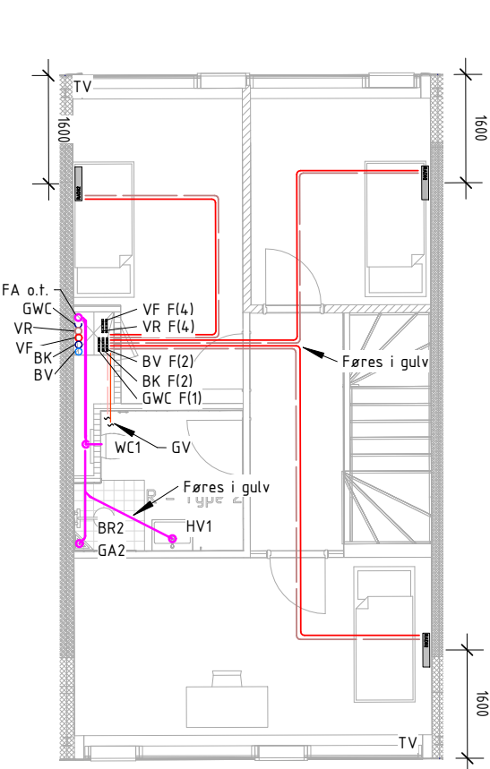
VVS ETAGE 02 Type R-3-C
