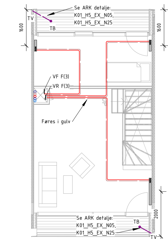
VVS ETAGE 01 Type R-3-G
