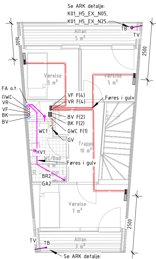
VVS ETAGE 02 Type R-3-B
