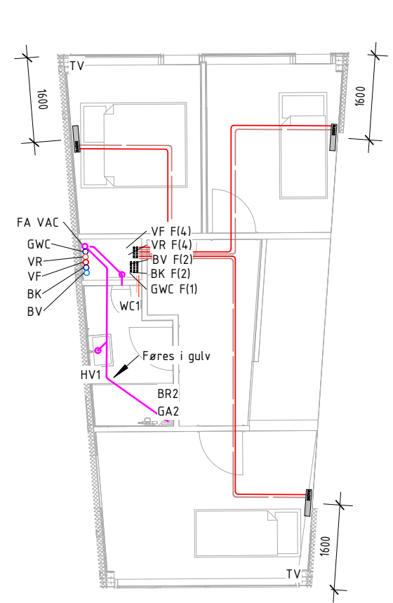
VVS ETAGE 02 Type R-3-F
