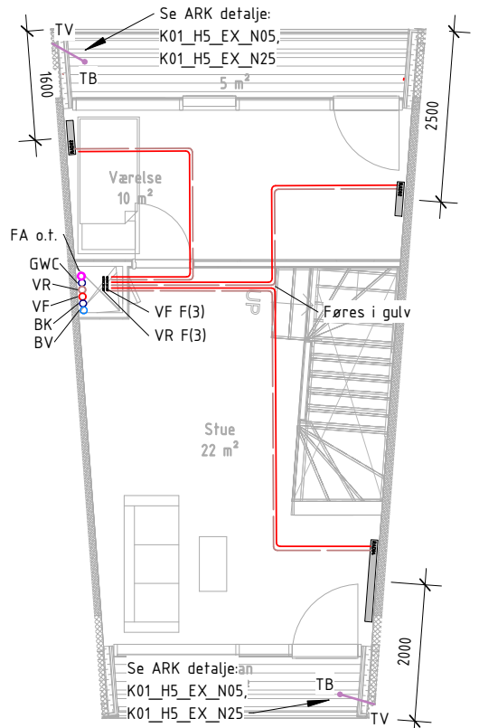
VVS ETAGE 01 Type R-3-A
