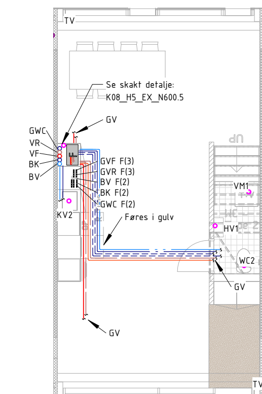
VVS ETAGE 00 Type R-3-G
