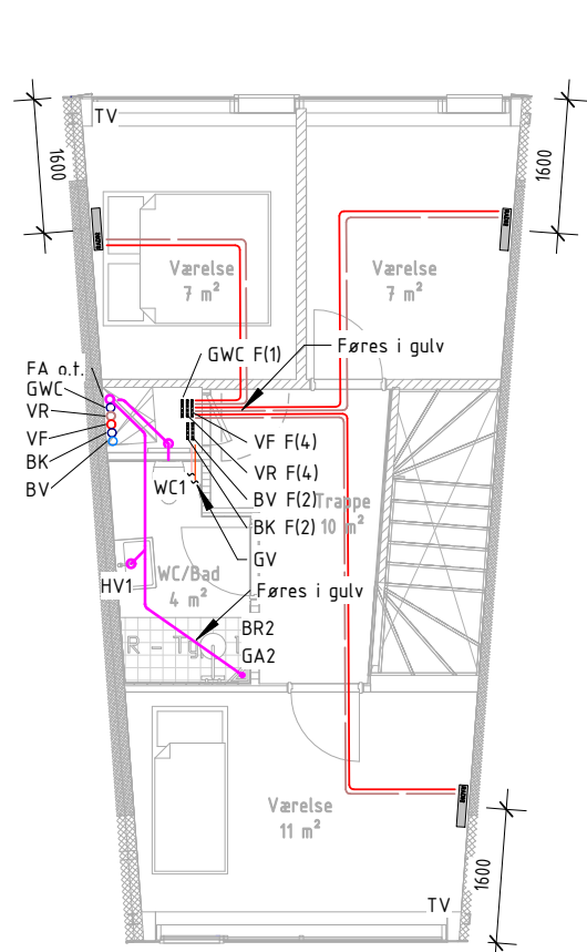
VVS ETAGE 02 Type R-3-A
