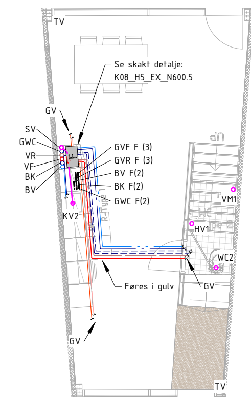
VVS ETAGE 00 Type R-3-F
