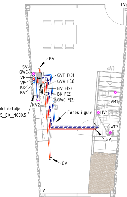
VVS ETAGE 00 Type R-3-E
