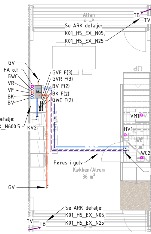
VVS ETAGE 00 Type R-3-D
