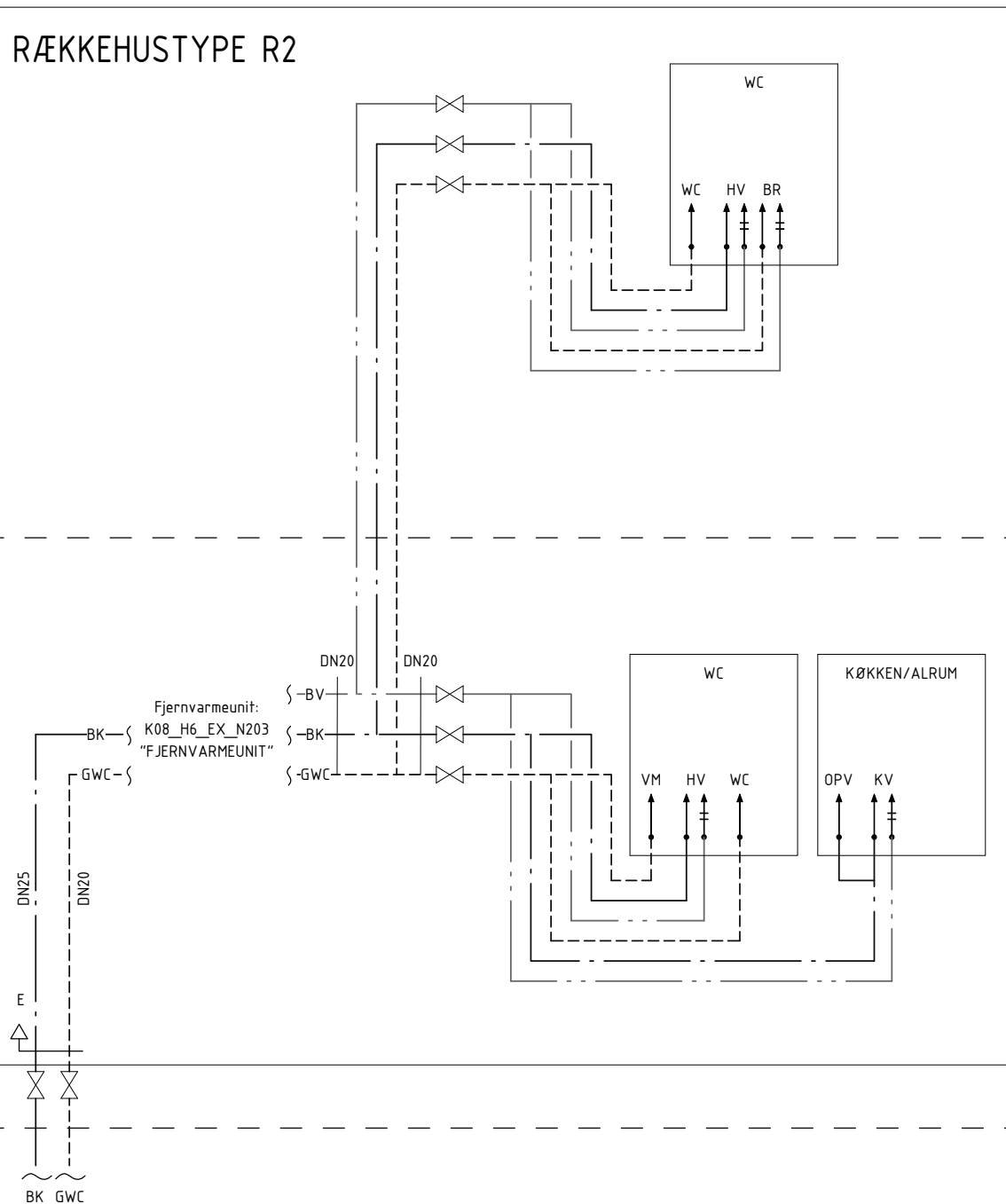
RÆKKEHUSTYPE R2
