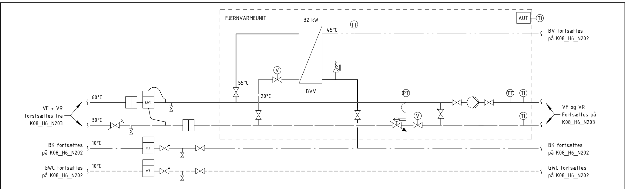
VARME - FJERNVARMEUNIT
